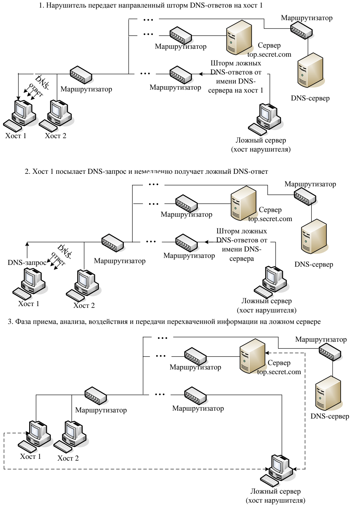
Рисунок 12. Схема реализации угрозы «внедрение ложного DNS-сервера»
